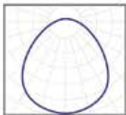
аксиальная КСС 90°
