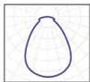
коэффициент КСС 80°
