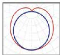
характеристики КСС 145°x115°
