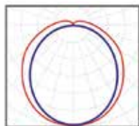
классическая КСС 110°
