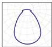
аксиальная КСС 60°
