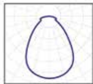
аксиальная КСС 60°
