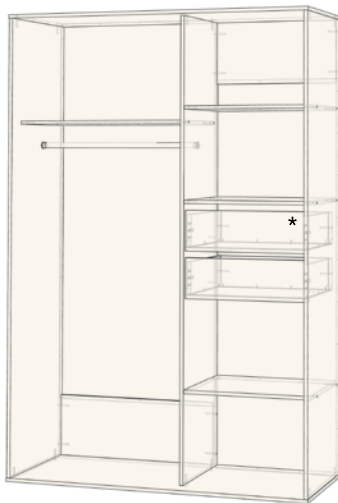
Компоновка шкафа шириной 120, 140 и 160 см
